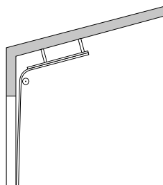
HLDU: Höhergeführter Laufschiene- Beschlag mit Dachfolge und unten- liegende Torsionsfederwelle
