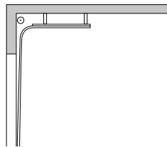
HL: Höhergeführter Laufschiene-Beschlag
