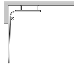
HLU: Höhergeführter Laufschiene- Beschlag mit untenliegender Torsionsfederwelle
