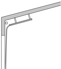
HLD: Höhergeführter Laufschiene- Beschlag mit Dachfolge (Maximale 30°)
